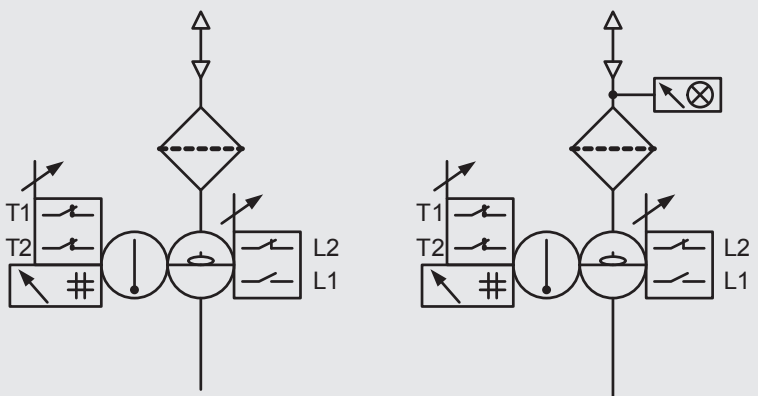
TC...W+D../-S12...
