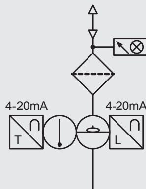
TC...UBM+C../-S44...
